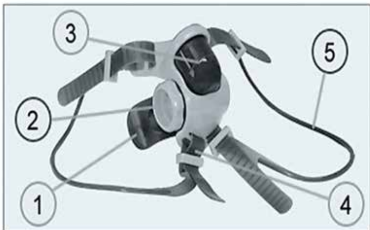
1 – корпус с загубником; 2 – нагрузочное устройство с ручками регуляции; 3 – клапан вдоха; 4 – держатель; 5 – крепежные ремни
